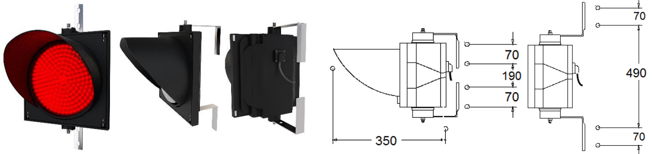
Beispiel-Abbildung LED-Ampel
