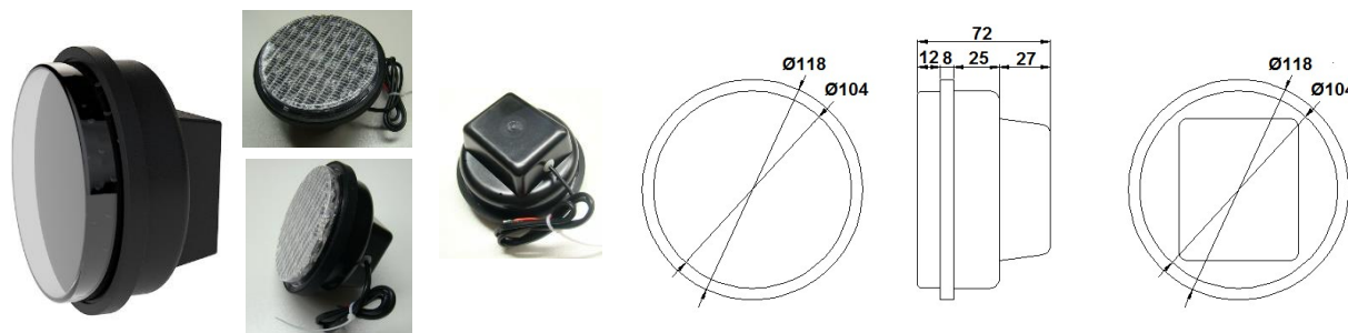
Beispiel-Abbildung LED-Ampel-Module
