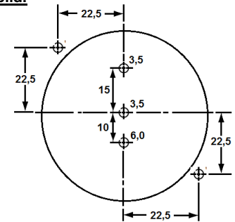
Bohrbild:
